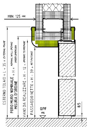
SEZ. A-A
