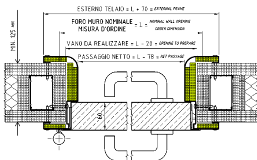
SEZ. B-B
